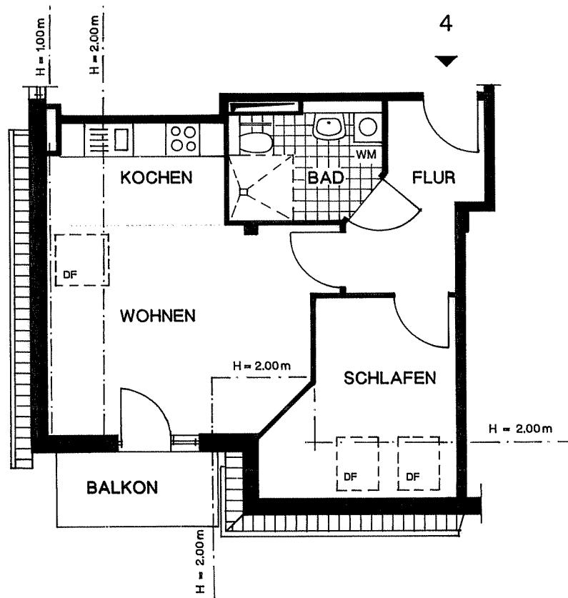
1. DACHGESCHOSS M 1:100
