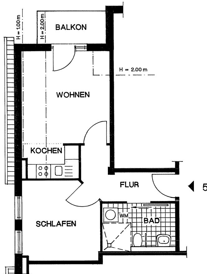
1. DACHGESCHOSS M 1:100
