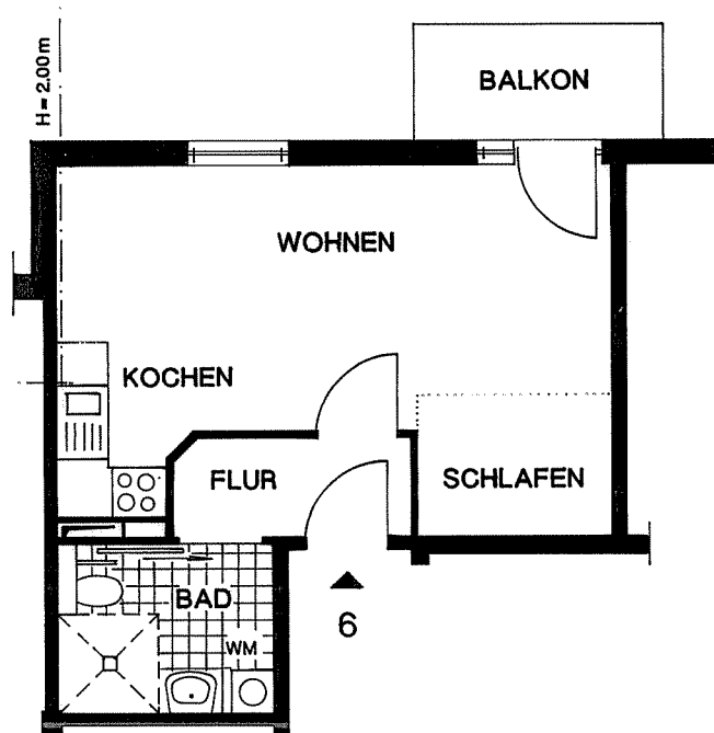
1. DACHGESCHOSS M 1:100
